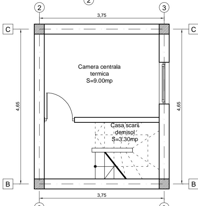
PLAN DEMISOL
