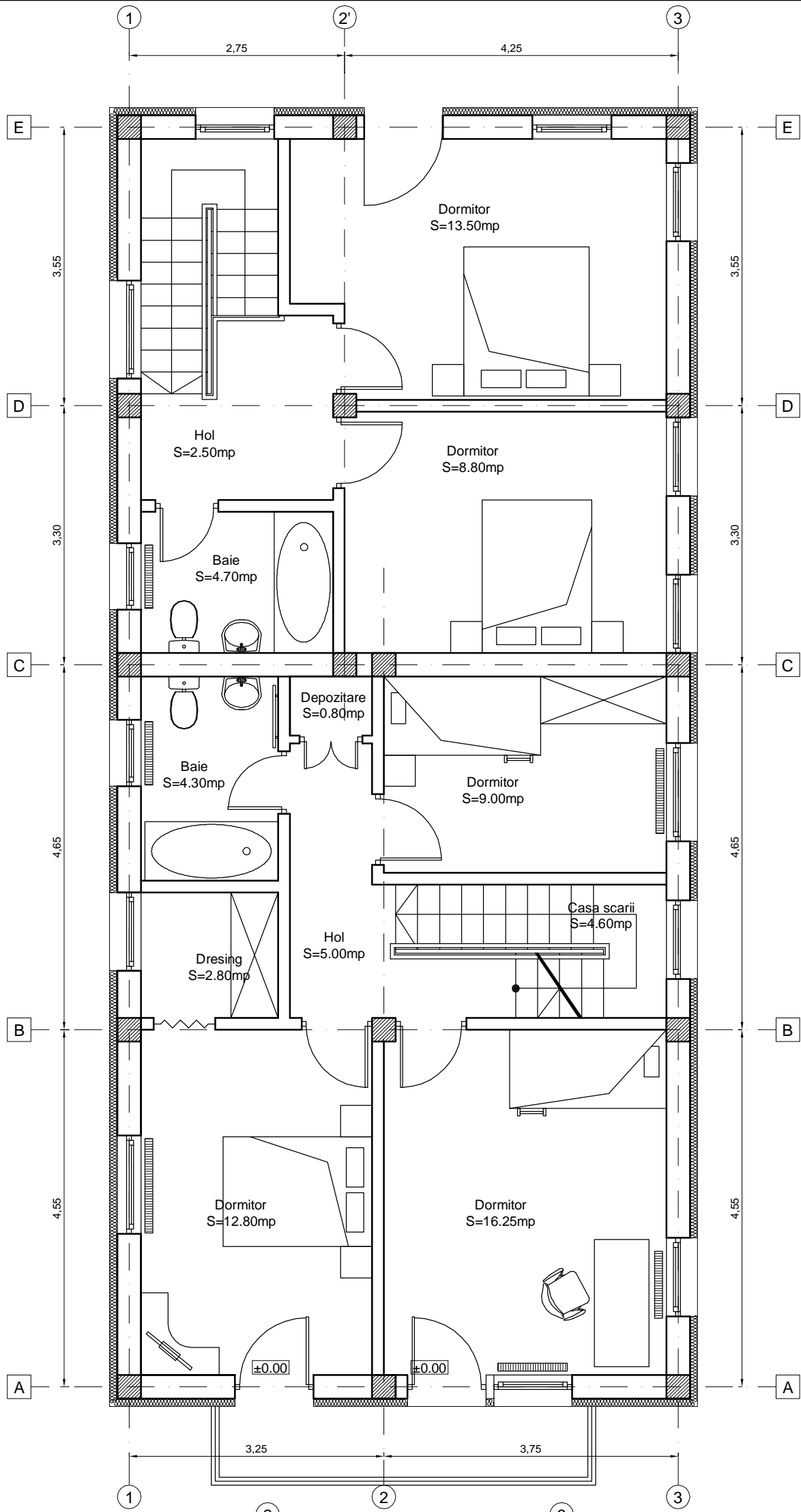
PLAN ETAJ
